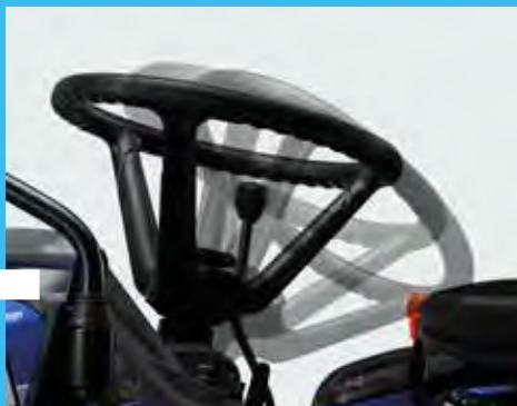
25°-ban dönthető kormányoszlop
